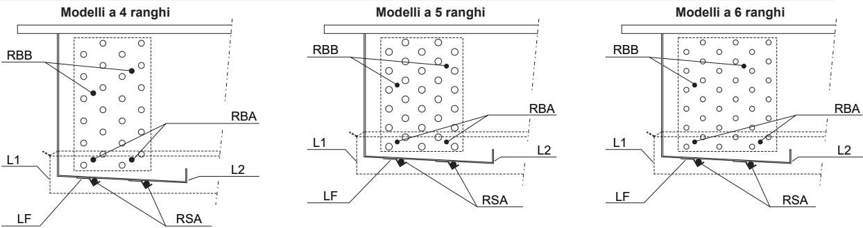
Particolare di posizionamento resistenze
