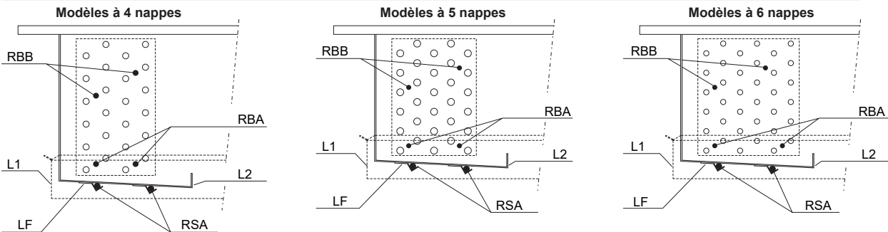
Détail de positionnement résistances électriques de dégivrage
