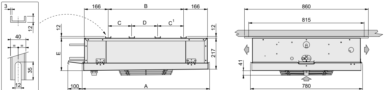
Detalle de la posición de las resistencias
