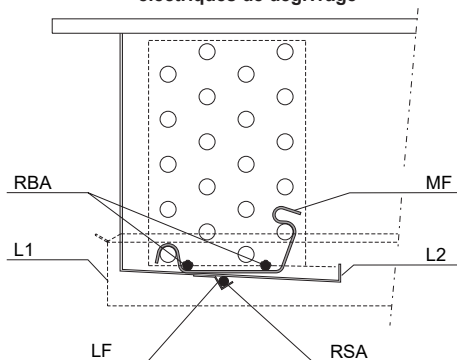
Détail de positionnement résistances électriques de dégivrage
