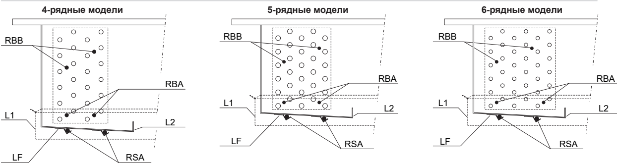
Расположением электрических ТЭНов оттайки
