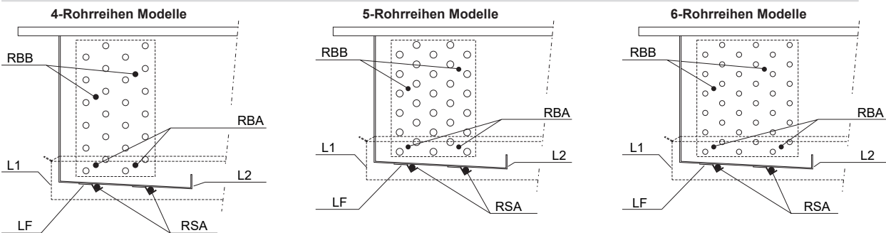
Einzelheit der Heizstäbebefestigung
