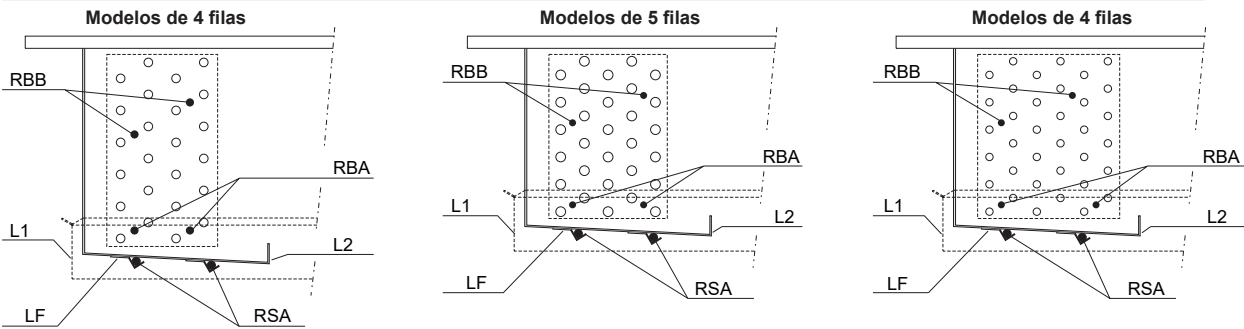
Detalle de la posición de las resistencias
