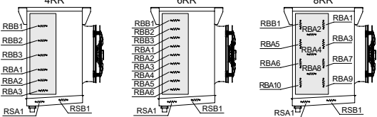
Particolari di posizionamento resistenze
