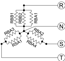
Conexión 400V/3/50-60Hz CONECTADO DE FÁBRICA
