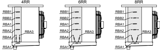
Détail de positionnement résistances
