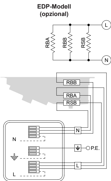
RBA - Hochleistungsheizstab im Wärmeaustauscher RBB - Niederleistungsheizstab im Wärmeaustauscher RSB - Hochleistungsheizstab in der inneren Tropfwanne
