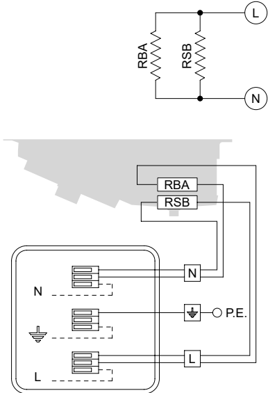
Стандартная модель
