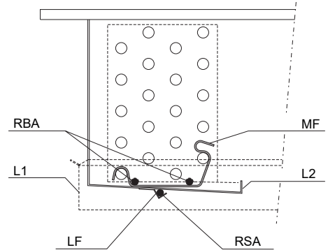
Расположением электрических ТЭНов оттайки
