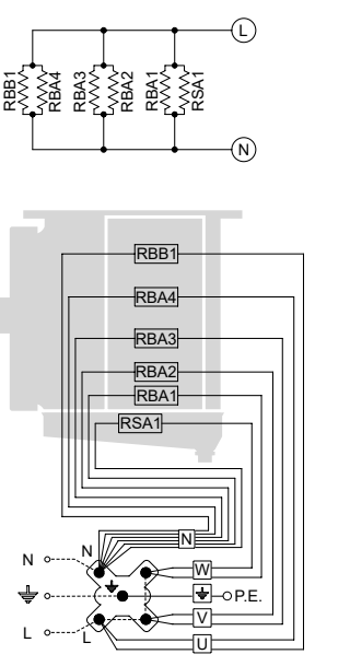
Anschluß 230V/1/50-60Hz vorzubereiten
