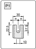
Détail de fixage
