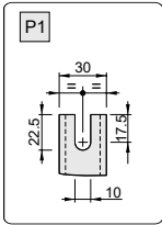
Einzelheit der Befestigung
