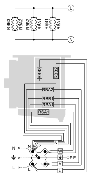
Connexion 230V/1/50-60Hz à predisposer
