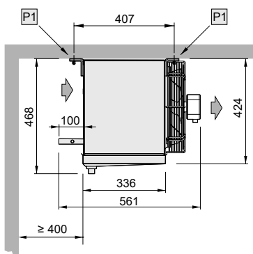
Détail de fixage
