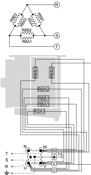
Подключение 230V/3/50-60Hz для подготовки
