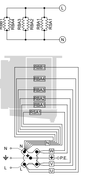
Connexion 230V/1/50-60Hz à predisposer
