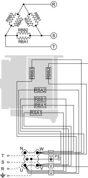
Conexión 230V/3/50-60Hz posible ver sistema
