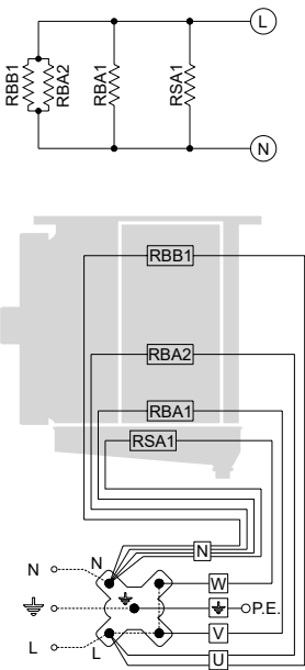
Connexion 230V/1/50-60Hz à prévoir
