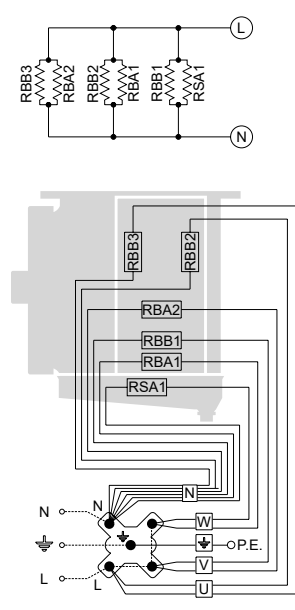
Anschluß 230V/1/50-60Hz vorzubereiten
