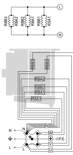
Подключение 230V/1/50-60Hz для подготовки
