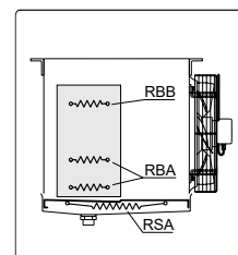
Détail de pos. résistances
