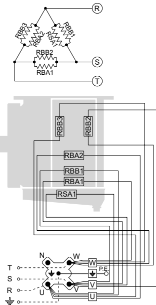
Connexion 230V/3/50-60Hz à predisposer
