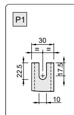
Détail de fixage
