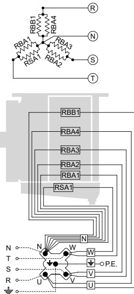
Connexion 400V/3/50-60Hz PRÉDISPOSÉE
