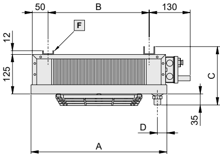
Particolare di posizionamento resistenze
