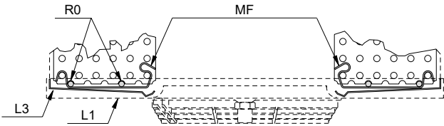
Particolare di posizionamento resistenze
