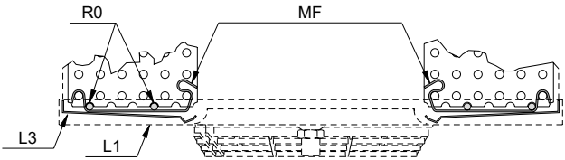
Einzelheit der heizstäbebefestigung
