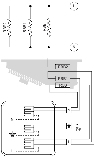
Collegamento modelli AGS4 L7 ED 230V/1/50-60Hz
