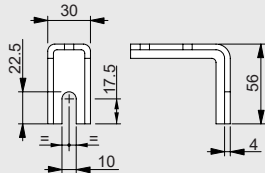
Detalle de fijación "Z"
