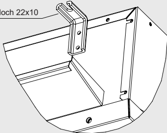
Einzelheit der Heizstäbebefestigung
