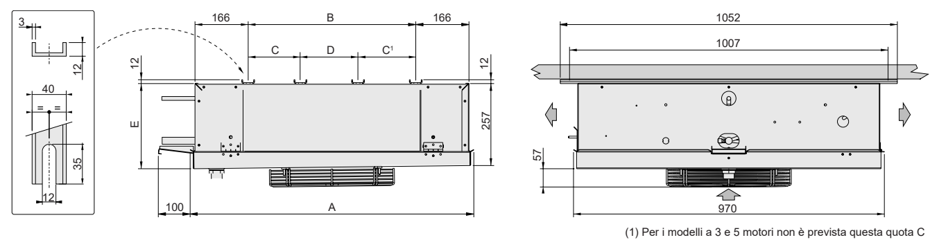
Particolare di fissaggio resistenze
