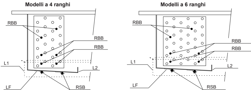
Particolare di fissaggio resistenze
