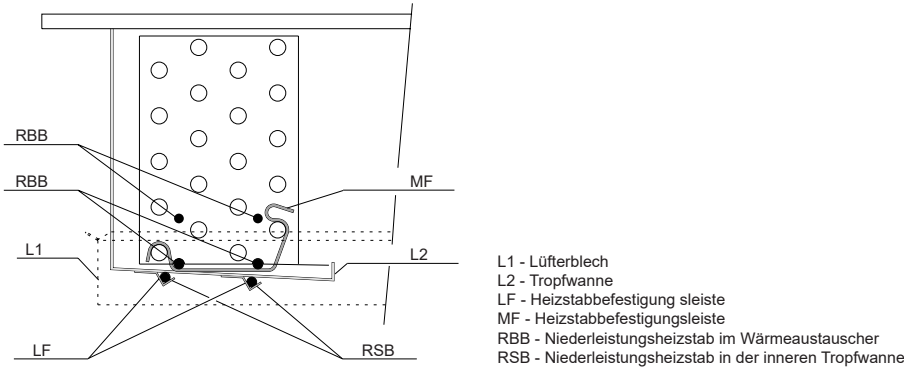
Einzelheit der Heizstäbebefestigung
