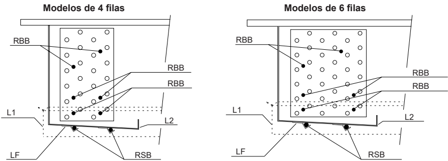
Detalle de la posición de las resistencias
