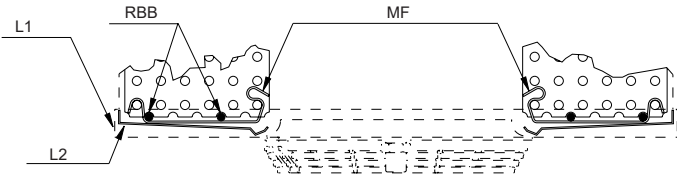
Einzelheit der Heizstäbebefestigung
