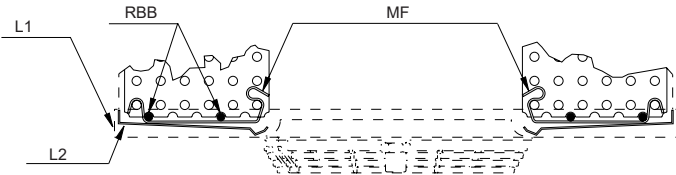
Détail de positionnement résistances électriques de dégivrage
