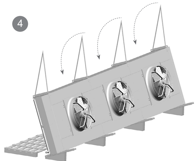
Colocar el modelo sobre la base inclinada
