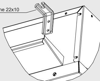
Détail de positionnement résistances
