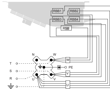
Подключение 230V/3/50-60Hz для подготовки
