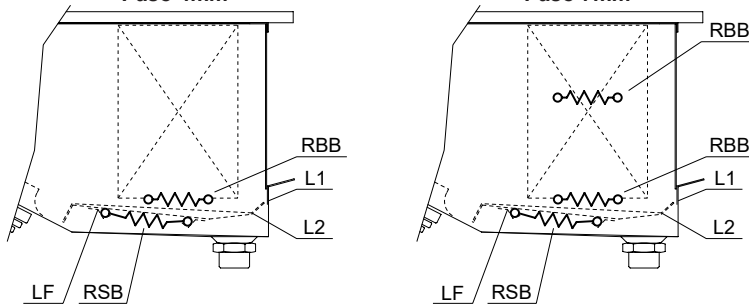
Detalle de la posición de las resistencias Paso 4mm Paso 7mm
