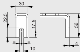
Деталь крепления "Z"
