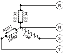
Collegamento 400V/3/50-60Hz PREDISPOSTO
