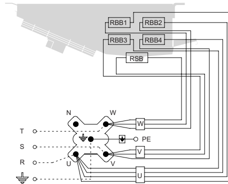
Collegamento 230V/3/50-60Hz da predisporre
