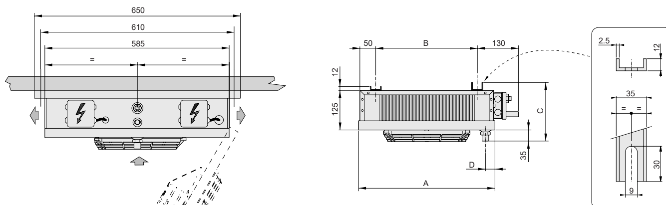
Расположением электрических ТЭНов оттайки
