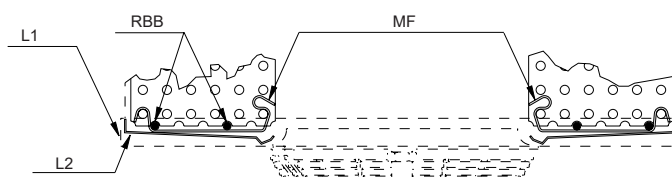
Einzelheit der Heizstäbefestigung
