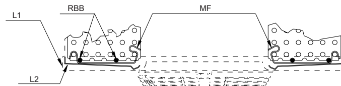
Расположением электрических ТЭНов оттайки
