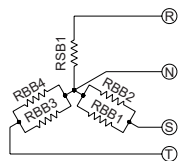
ПОДКЛЮЧЕНИЕ 400V/3/50-60Hz подготовлено
