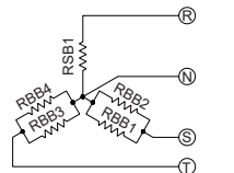
Connexion 400V/3/50-60Hz PRÉDISPOSÉE
