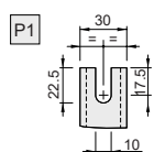
Деталь крепления
