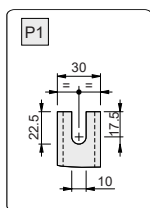
Деталь крепления
