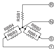
Conexión 400V/3/50-60Hz CONECTADO DE FÁBRICA
