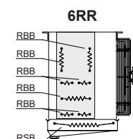
Detalle de la posición de las resistencias
