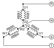
Anschluß 400V/3/50-60Hz STANDARD
