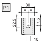
Détail de fixation
