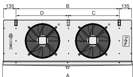
Detalle de fijación
