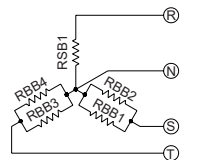
Collegamento 400V/3/50-60Hz PREDISPOSTO
