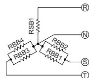
Anschluß 400V/3/50-60Hz STANDARD
