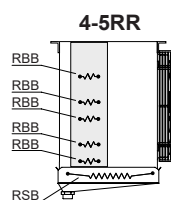
Detalle de la posición de las resistencias
