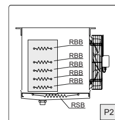
P1: Деталь крепления P2: Детальное расположение ТЭНов
