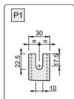
Détail de fixage
